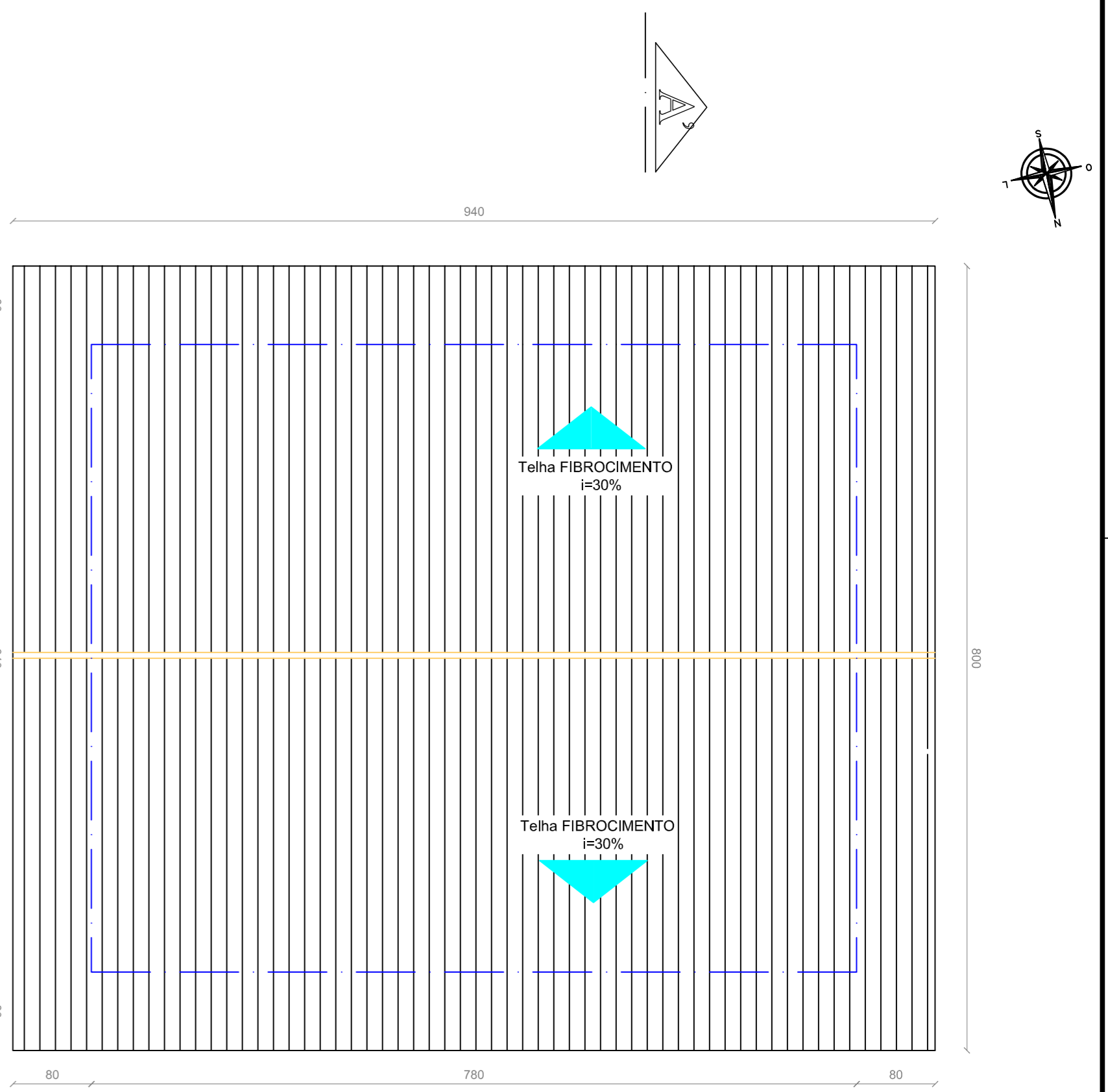
PLANTA COBERTURA Escala: 1/50
