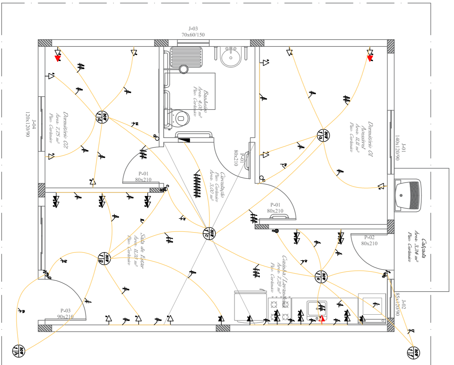
ELETRICO Escala: 1/50
