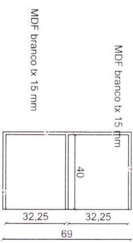
Corte BB
