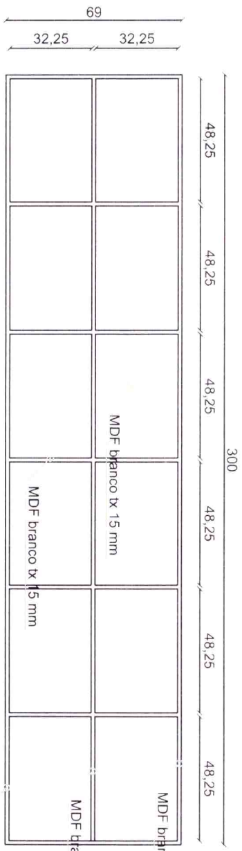
Corte AA
